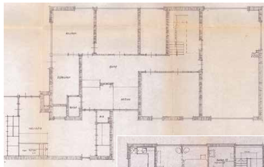
Tekeningen van de herinrichting van de begane grond en eerste verdieping bij het vertrek van de zusters
