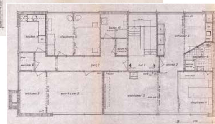
Tekeningen van de herinrichting van de begane grond en eerste verdieping bij het vertrek van de zusters
